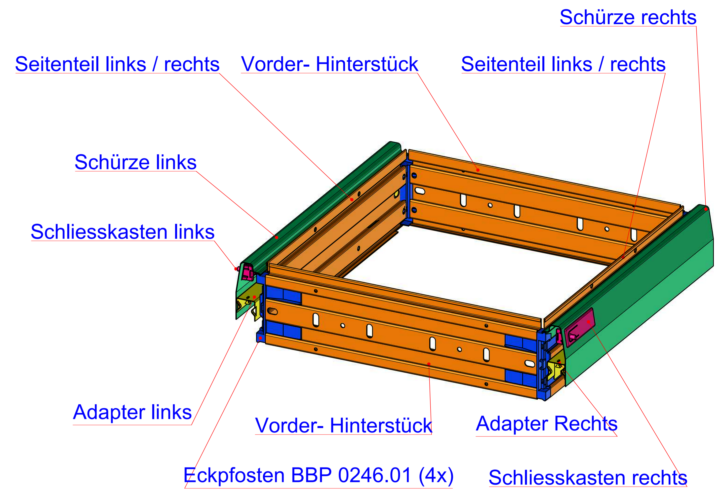
Isometrische Ansicht M 1:2
